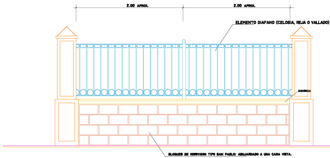
ALZADO
