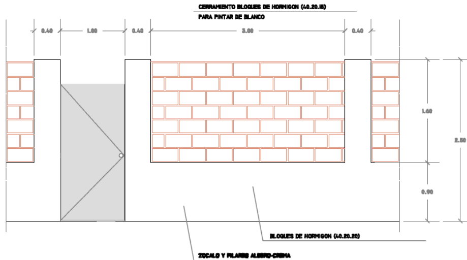
ALZADO
