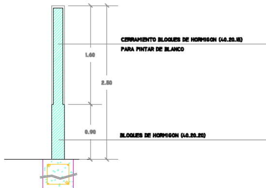
SECCION
