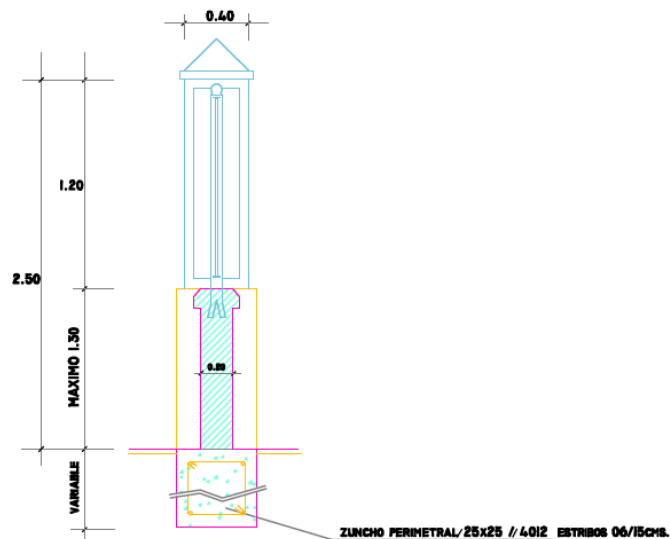
SECCION
